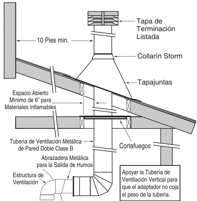
Figura 12. – Instalación Típica de la Tubería del Ventilador Metálico - EE.UU. (Presión Negativa - Vertical)
