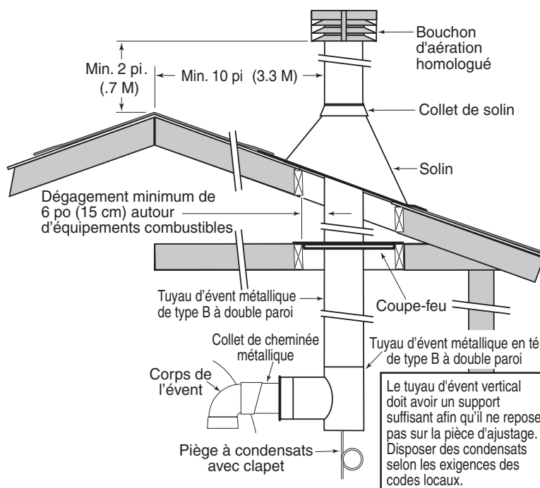
Figure 13. – L'installation de tuyau de conduit en métal typique - Canada. (Verticale- la Pression Négative)
