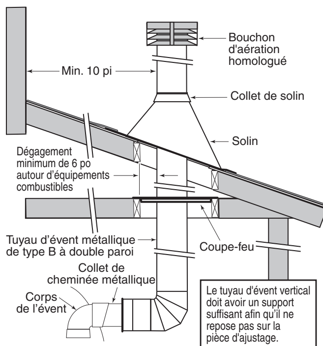
Figure 12. – L'installation de tuyau de conduit en métal typique - É.-U. (Verticale- la Pression Négative)
